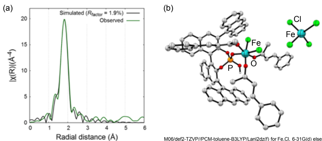
図 1. (a) Fe K-edge in situ XAFS 測定 (b) 密度汎関数理論により求めた推定溶液構造
