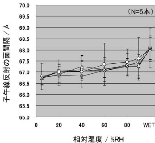
図1. 加湿に伴う子午線反射の面間隔変化
