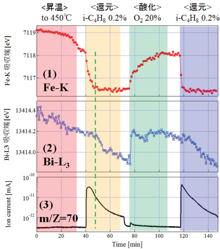
Fig.2. (1)Fe-K 端の吸収端シフトの時間変化 (2)Bi-L III 端の吸収端シフトの時間変化 (3)m/Z=70(メタクロレイン親イオン)のイオン電流の時間変化(ガスフロー過程をそろえて表示させた。)
