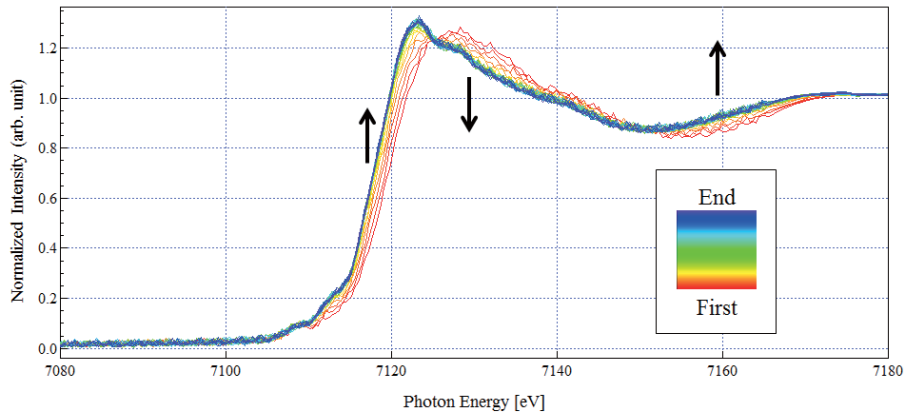
Fig.1. Fe-K 端 還元過程のスペクトル変化(赤→青)
